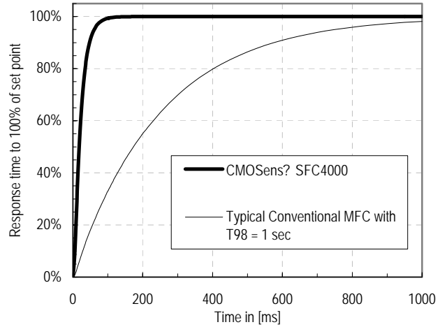
图 4: SFC4000 响应时间
