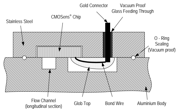
图 8: 真空玻璃密封截面图（纵切面）
