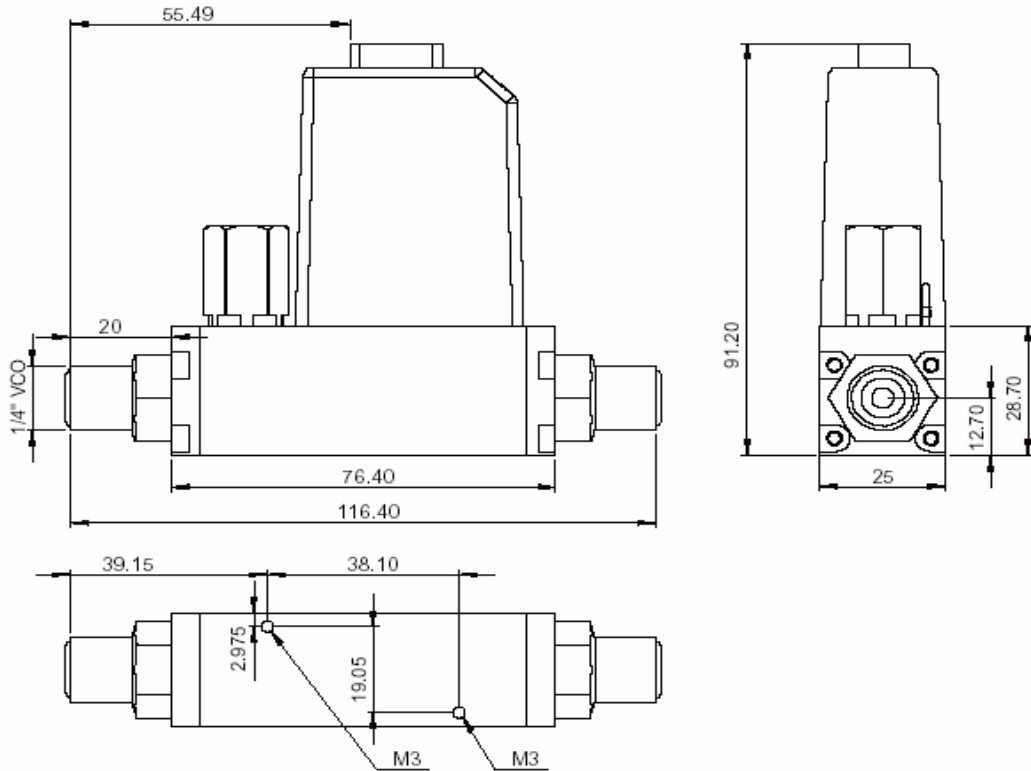
图 32: 1/4" VCO 模式物理尺寸和包装信息. 单位 [mm]
