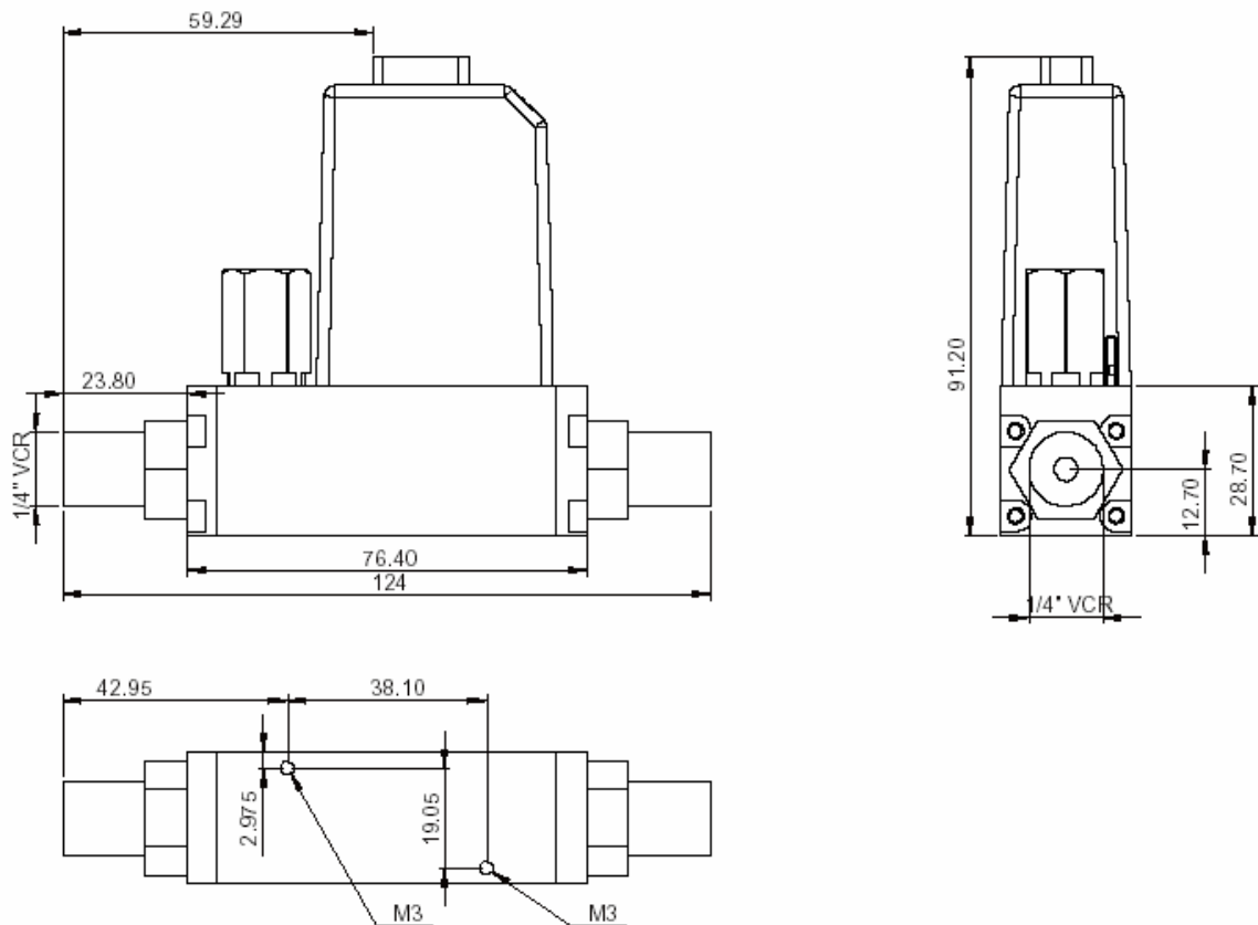
图 43: 1/4" VCR 模式物理尺寸和包装信息. 单位 [mm]
