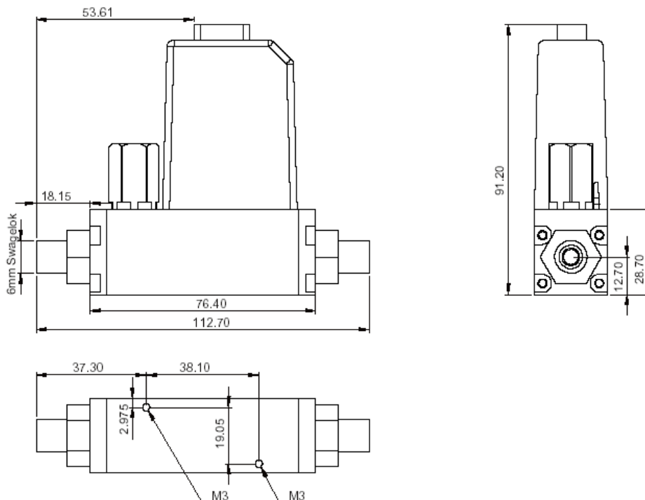
图 21: 6mmSwagelok 物理尺寸和包装信息. 单位 [mm]
